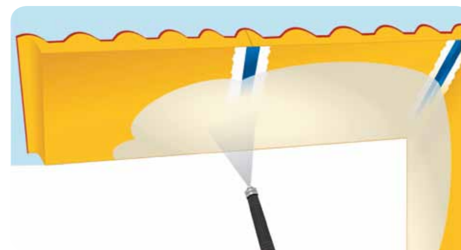
Applicazione di Sigilpanel lungo la giunzione di due pannelli mediante rinforzo con Hydroflex bandella.
